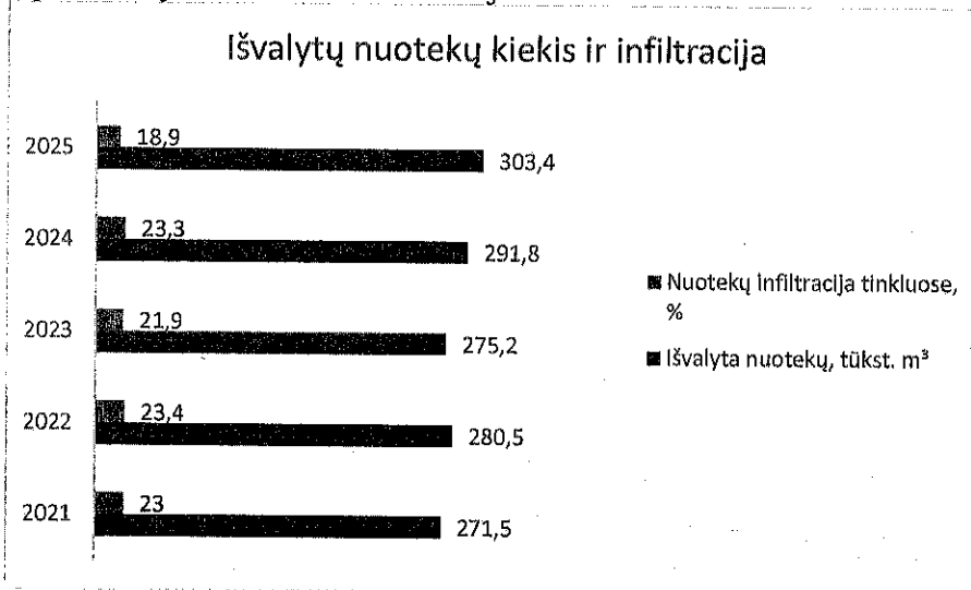
4 pav. Išvalytos nuotekos ir infiltracija
