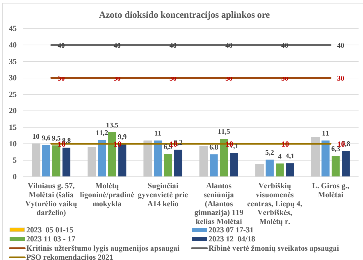
1.8.2 pav. NO 2 tyrimų duomenys Molėtų r. savivaldybė 2023 m. aplinkos oro monitoringo vietose
