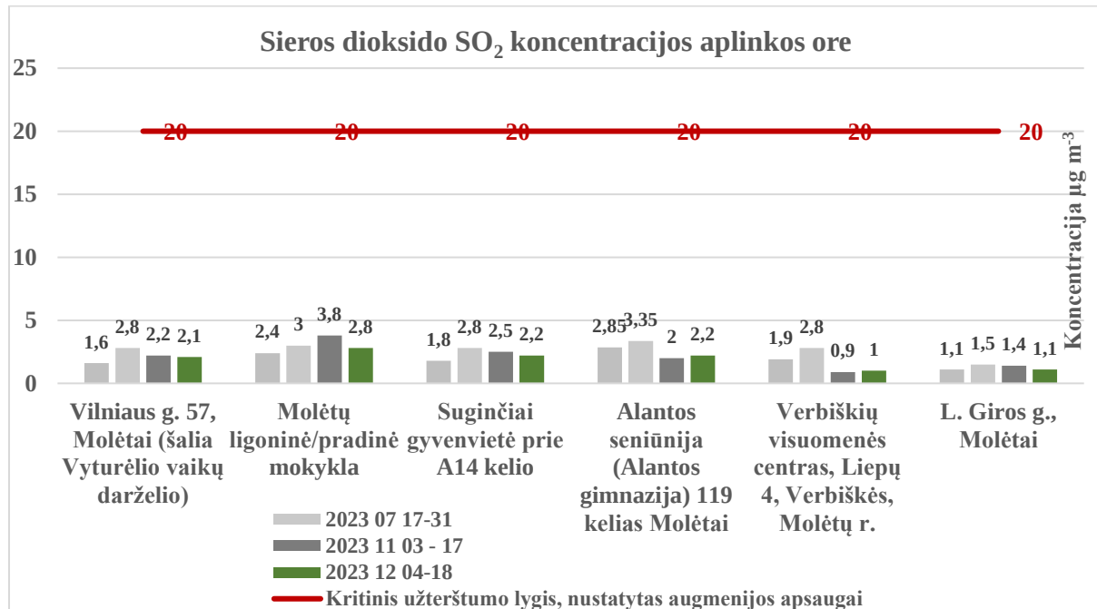
1.8.4 pav. Sieros dioksido (SO 2 ) koncentracijos reikšmės 2023 m. Molėtų r. aplinkos oro monitoringo vietose
