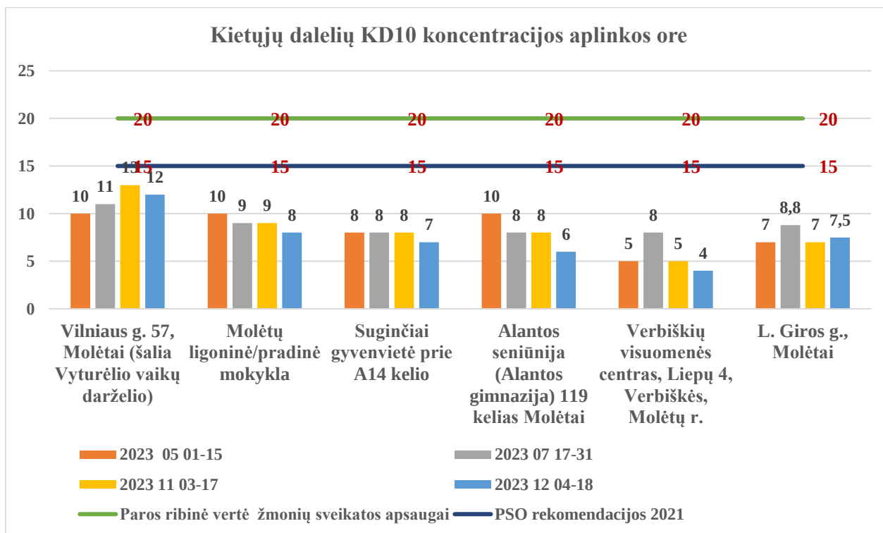
1.8.3.1 pav. Kietųjų dalelių KD 10 koncentracijos 2023 m. Molėtų r. oro monitoringo vietose
