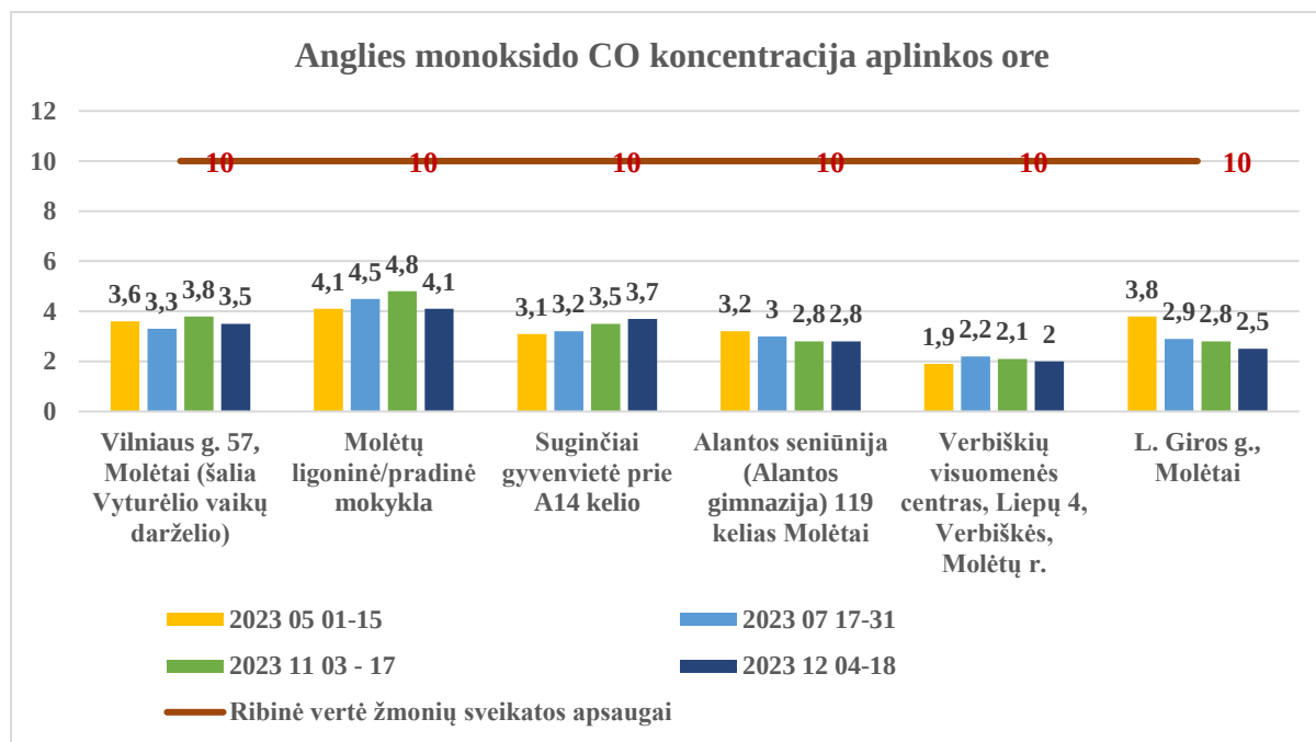
1.8.5 pav. Nustatytos anglies monoksido CO koncentracijos 2023 m. Molėtų r. tiriamaisiais laikotarpiais.
