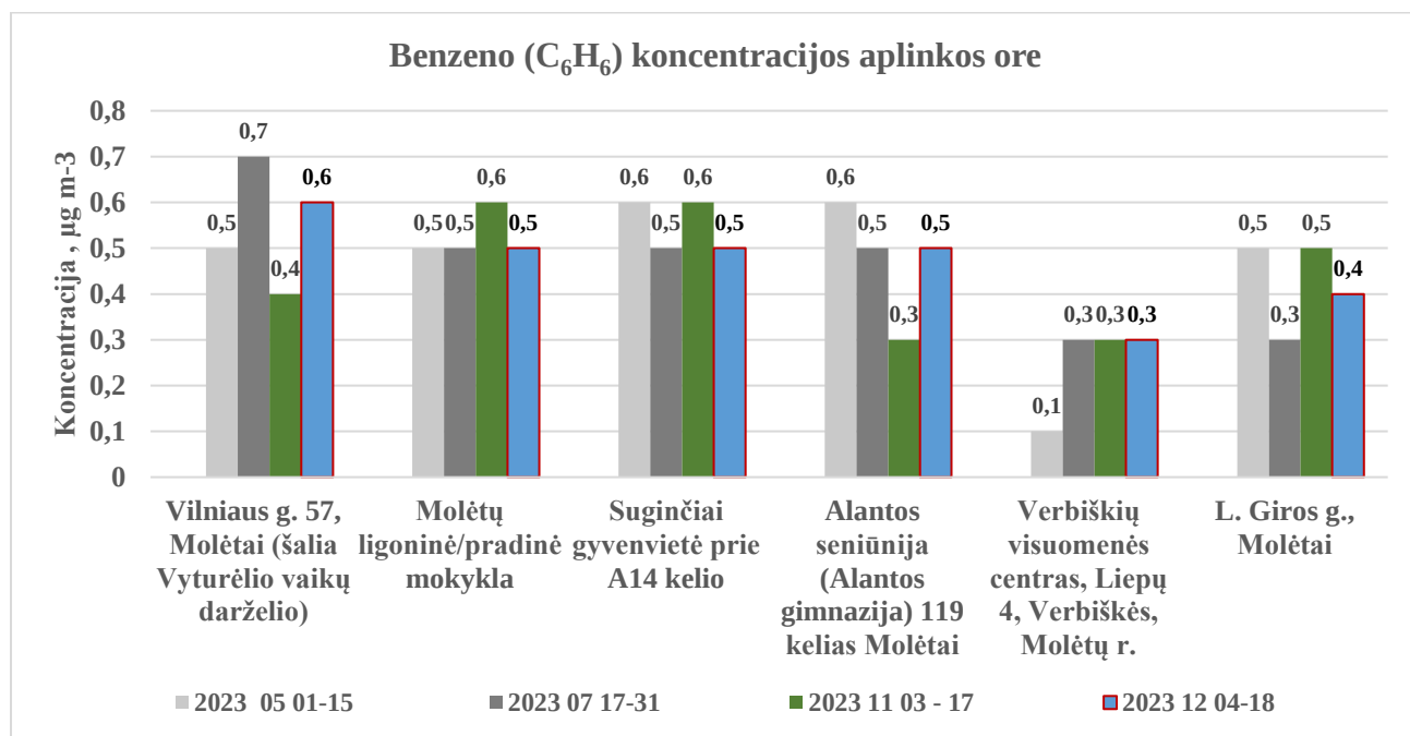
1.8.5 pav. Nustatytos benzeno C 6 H 6 koncentracijos 2023 m. Molėtų r. tiriamaisiais laikotarpiais
