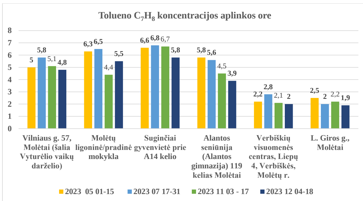
1.8.7 pav. Nustatytos tolueno (C 7 H 8 ) koncentracijos 2023 m. Molėtų r. tiriamaisiais laikotarpiais
