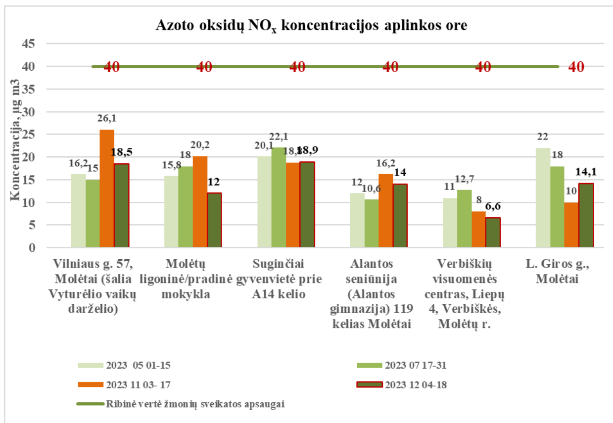
1.8.1 pav. NO x tyrimų duomenys Molėtų r. savivaldybė aplinkos oro monitoringo vietose 2023 m.
