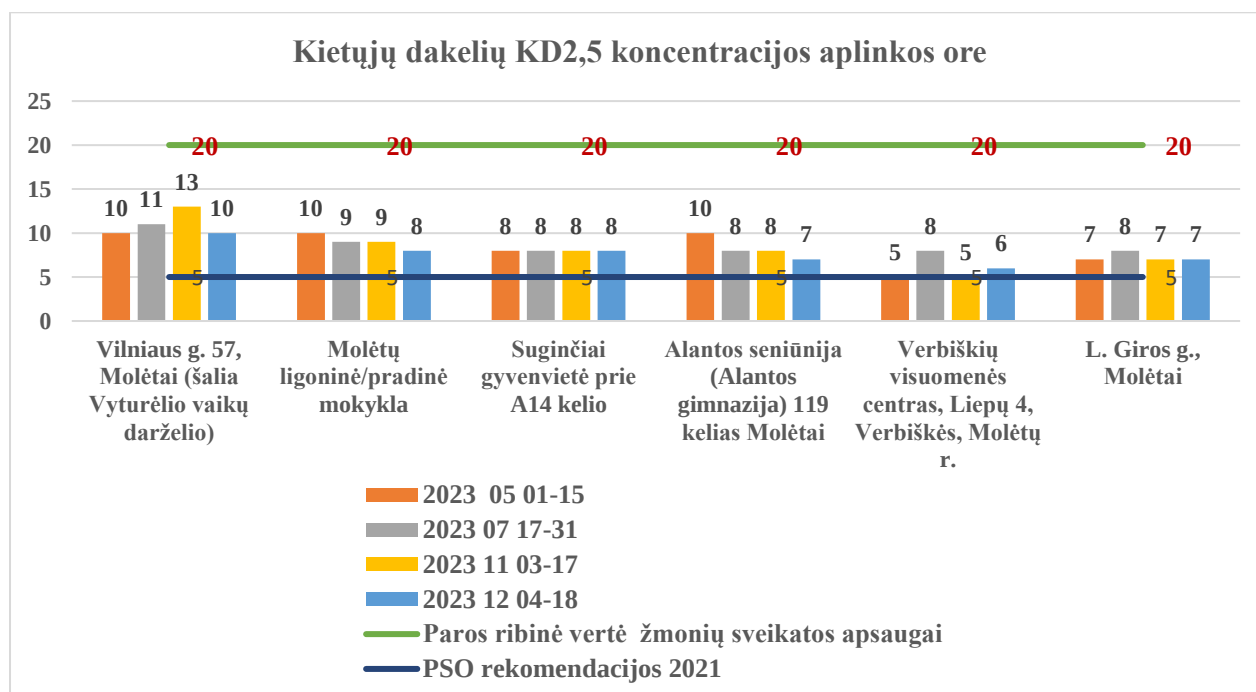
1.8.3.2 pav. Kietųjų dalelių KD 2,5 koncentracijos 2023 m. Molėtų r. oro monitoringo vietose
