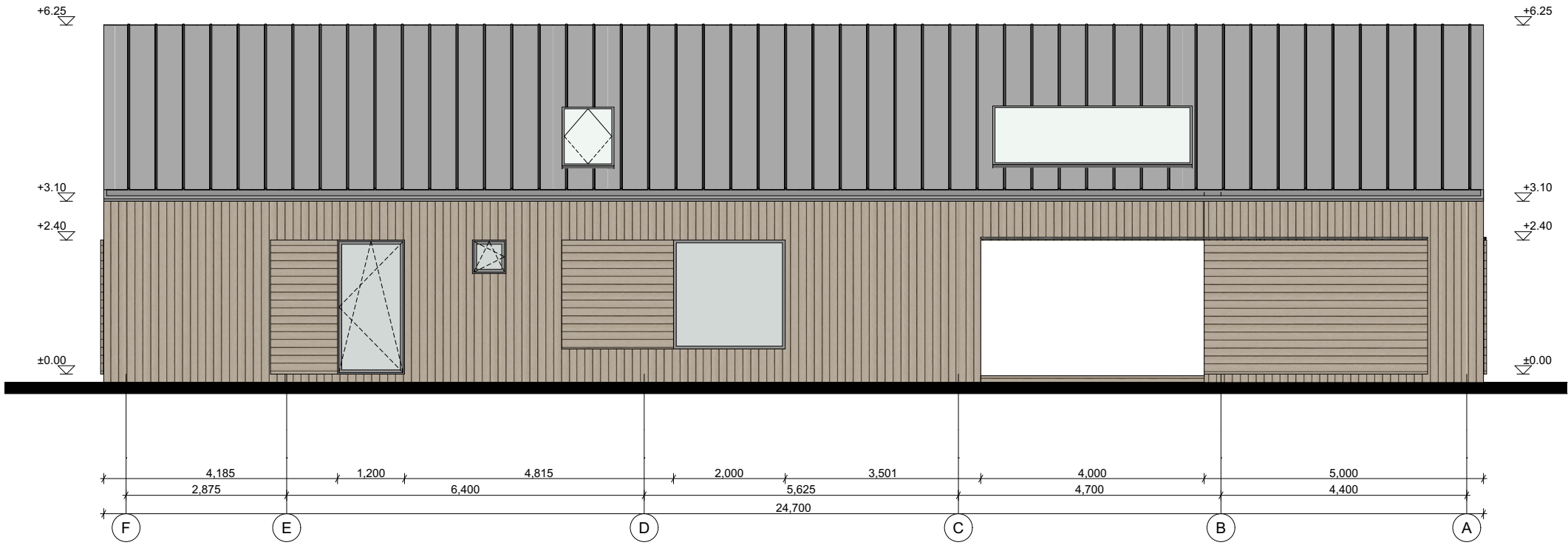
Vakarų fasadas
