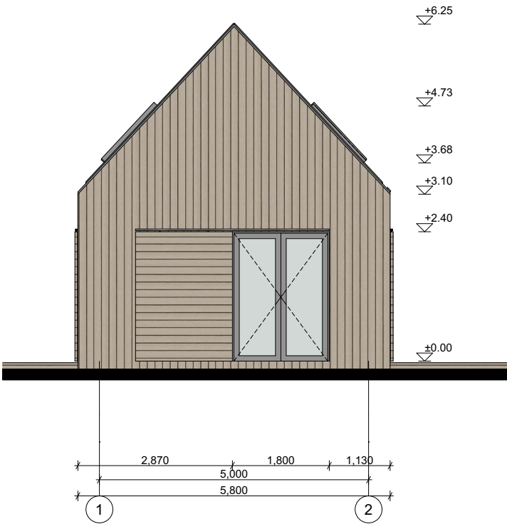
Pietų fasadas
