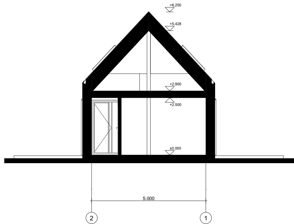
A Pjūvis A-A 1:100
