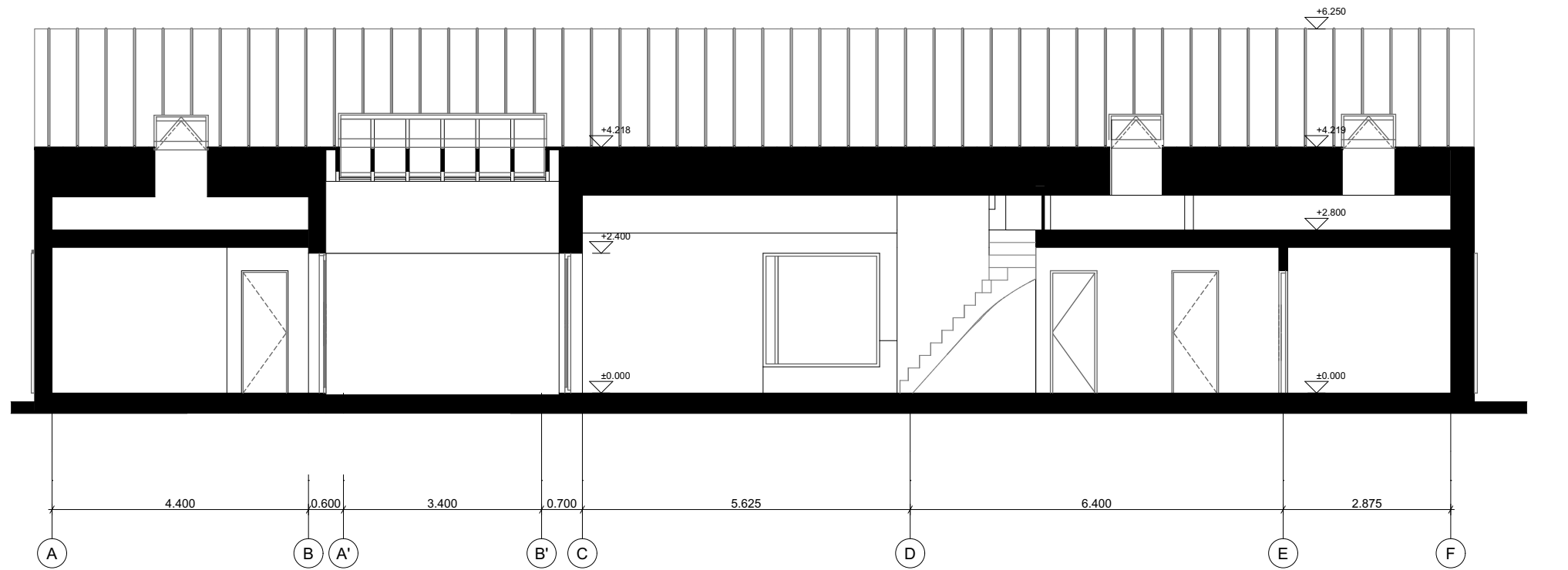
C Pjūvis C-C 1:100
