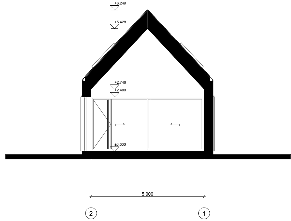
B Pjūvis B-B 1:100
