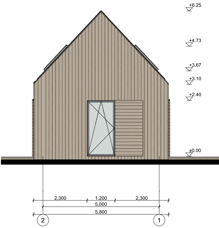
Šiaurės fasadas
