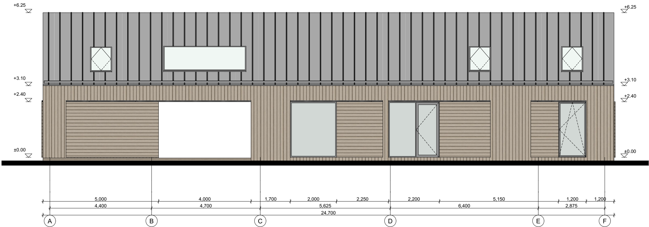
Rytų fasadas
